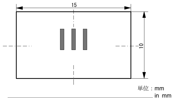
第2図 たわみ試験用プリント基板 Figure 2. PCB for Bending Strength Test
