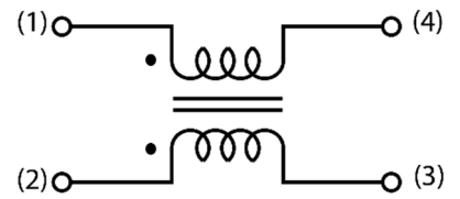
■等価回路図
