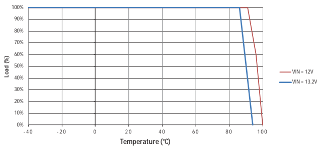
MGJ2D121509MPC
