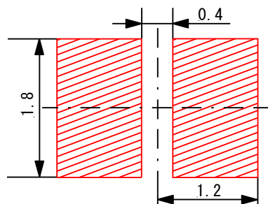
(推奨ランド寸法) (Recommendable Land Pattern)
