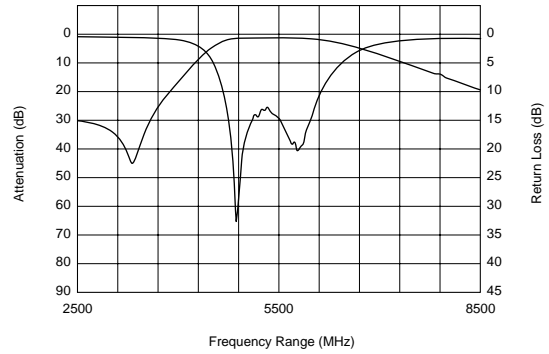
周波数特性データ
