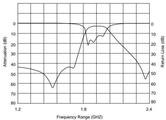
周波数特性データ
