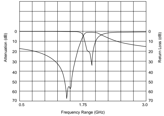
周波数特性データ
